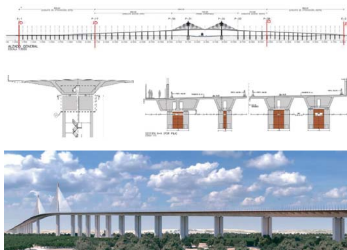
Diferentes secciones incluidas en el proyecto y el diseño general que se pretende conseguir. MITMA
